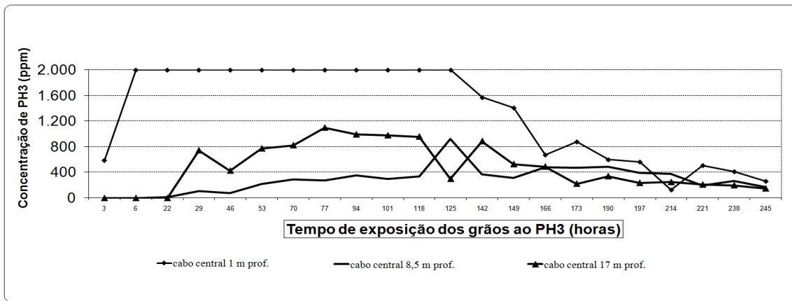
FIGURA 1. Monitoramento da concentração da fosfina ( \text{PH}_3 ) medida em diferentes profundidades, durante o expurgo em silo metálico de 9.400 t, com distribuição das pastilhas de fosfina na superfície da massa de grãos sem circulação da fosfina. Coamo, Arapuã, PR, 2016.
