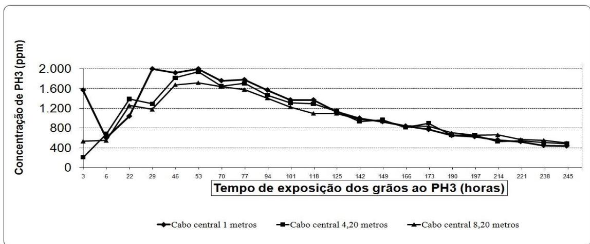
FIGURA 9. Monitoramento da concentração da fosfina (PH 3 ) medida em diferentes profundidades, durante o expurgo em armazém/célula de 1.100 t, com distribuição das pastilhas de fosfina na superfície da massa de grãos com o sistema de recirculação da fosfina. Coamo, Manoel Ribas, PR, 2016.
