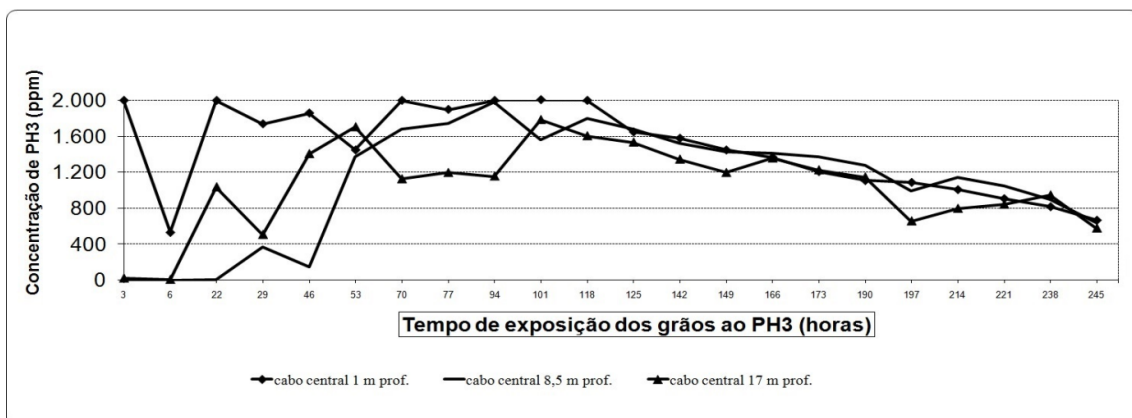
FIGURA 3. Monitoramento da concentração da fosfina ( \text{PH}_3 ) medida em diferentes profundidades, durante o expurgo em silo metálico de 9.400 t, com distribuição das pastilhas de fosfina na superfície da massa de grãos com o sistema de recirculação da fosfina. Coamo, Arapuã, PR, 2016.
