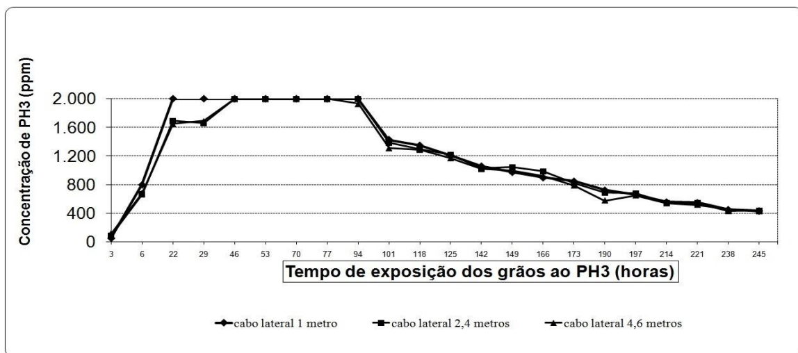
FIGURA 8. Monitoramento da concentração da fosfina (PH 3 ) medida em diferentes profundidades, durante o expurgo em armazém/célula de 1.100 t, com distribuição das pastilhas de fosfina na superfície da massa de grãos com o sistema de recirculação da fosfina. Coamo, Manoel Ribas, PR, 2016.
