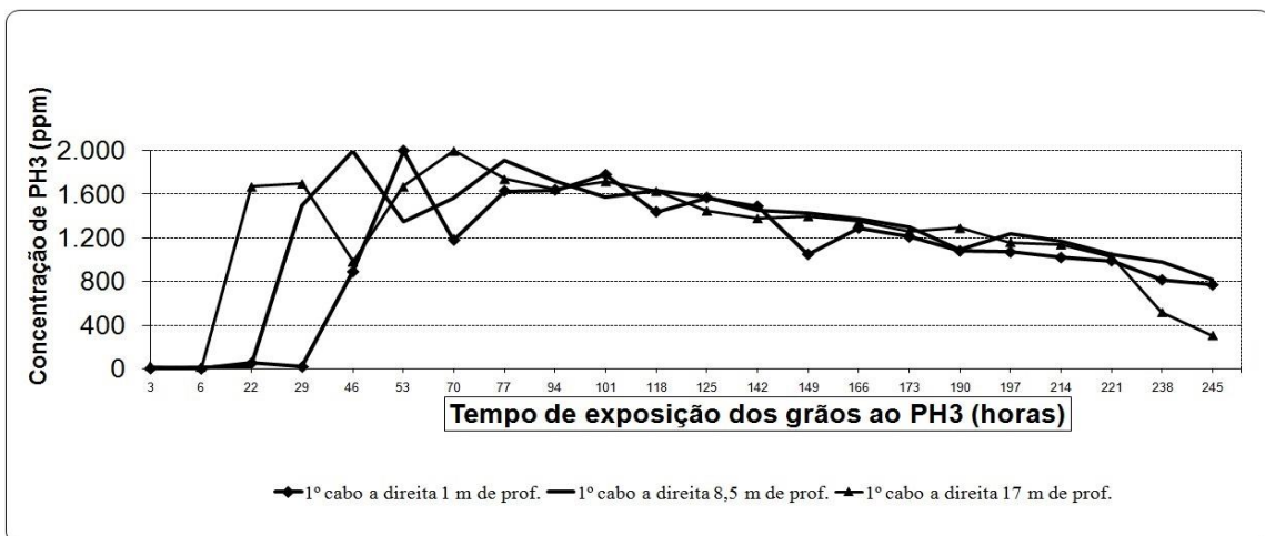
FIGURA 5. Monitoramento da concentração da fosfina (PH 3 ) medida em diferentes profundidades, durante o expurgo em silo metálico de 9.400 t, com distribuição das pastilhas de fosfina na superfície da massa de grãos com o sistema de recirculação da fosfina. Coamo, Arapuã, PR, 2016.
