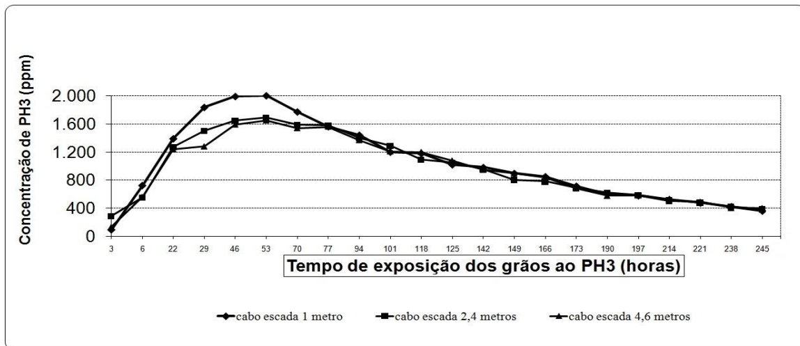
FIGURA 7. Monitoramento da concentração da fosfina (PH 3 ) medida em diferentes profundidades, durante o expurgo em armazém/célula de 1.100 t, com distribuição das pastilhas de fosfina na superfície da massa de grãos sem o sistema de recirculação da fosfina. Coamo, Manoel Ribas, PR, 2016.
