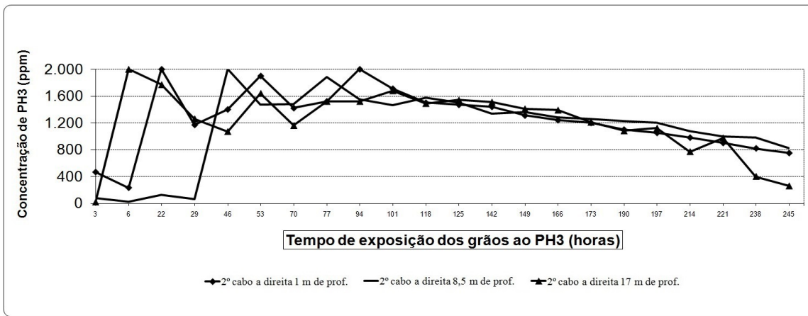
FIGURA 4. Monitoramento da concentração da fosfina (PH 3 ) medida em diferentes profundidades, durante o expurgo em silo metálico de 9.400 t, com distribuição das pastilhas de fosfina na superfície da massa de grãos com o sistema de recirculação da fosfina. Coamo, Arapuã, PR, 2016.
