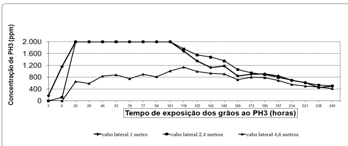
FIGURA 6. Monitoramento da concentração da fosfina (PH 3 ) medida em diferentes profundidades, durante o expurgo em armazém/célula de 1.100 t, com distribuição das pastilhas de fosfina na superfície da massa de grãos sem o sistema de recirculação da fosfina. Coamo, Manoel Ribas, PR, 2016.
