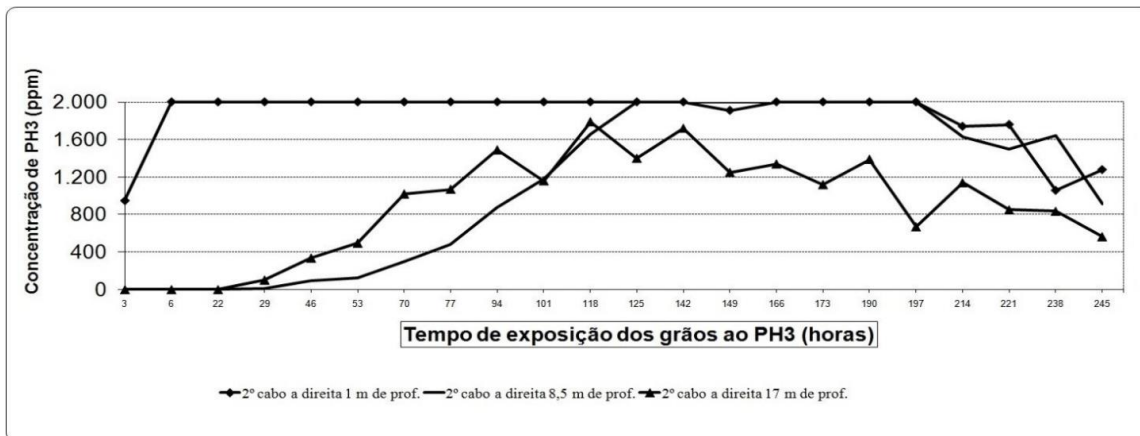
FIGURA 2. Monitoramento da concentração da fosfina ( \text{PH}_3 ) medida em diferentes profundidades, durante o expurgo em silo metálico de 9.400 t, com distribuição das pastilhas de fosfina na superfície da massa de grãos sem circulação da fosfina. Coamo, Arapuã, PR, 2016.
