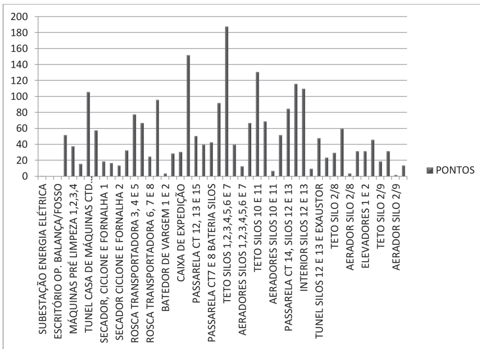
FIGURA 4. Número de insetos-praga, por ponto de monitoramento do Manejo Integrado de Pragas na Unidade Armazenadora de Toledo, PR.
