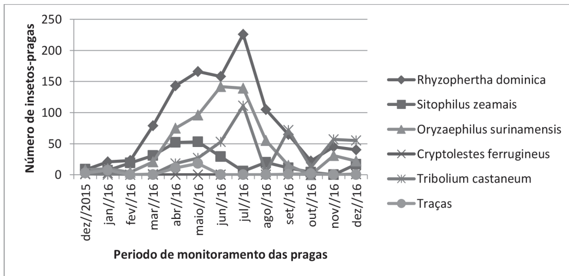
FIGURA 2. Número de insetos-praga, ao longo dos 13 meses de armazenamento dos grãos, encontrados durante o monitoramento do Manejo Integrado de Pragas na Unidade Armazenadora de Toledo, PR.
