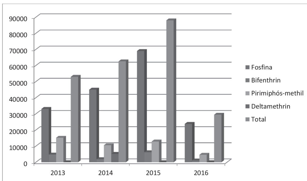
FIGURA 5. Relação dos custos de tratamento com inseticidas, massa de grãos e estrutura. Usados na unidade armazenadora de Toledo, ao longo dos últimos quatro anos.
