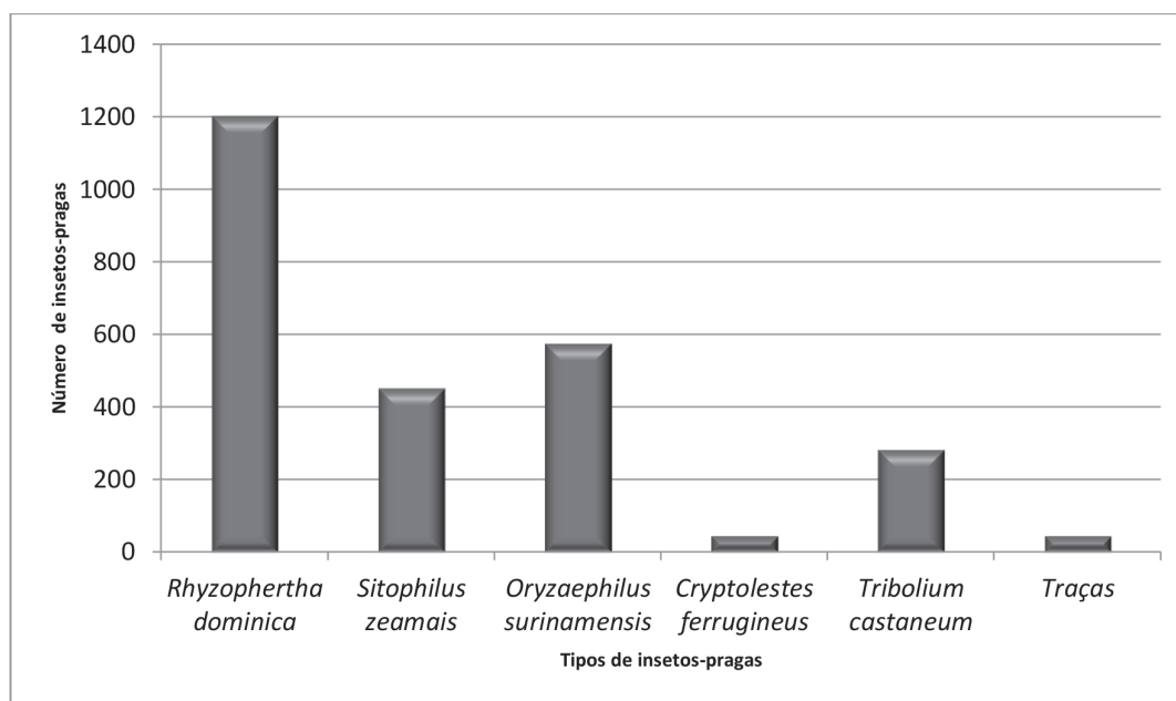
FIGURA 3. Número de insetos-praga, por espécie, ao longo dos 13 meses de armazenamento dos grãos, encontrados durante o monitoramento do Manejo Integrado de Pragas na Unidade Armazenadora de Toledo, PR.
